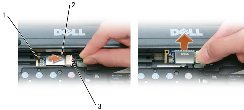
1 金属卡舌 2 插卡 3 电缆连接器
