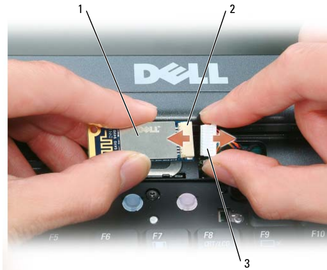
1 插卡 2 插卡连接器 3 电缆连接器
